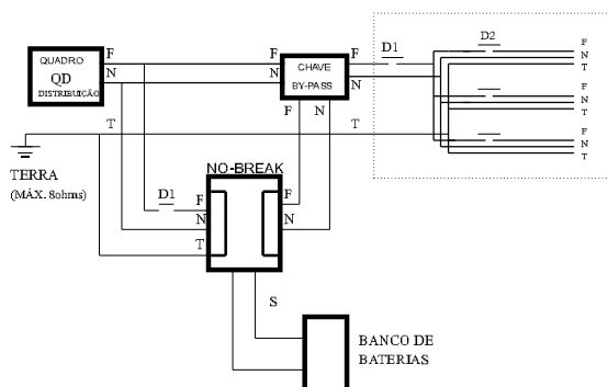
Figura 3 - Instalação Elétrica com chave By-P
